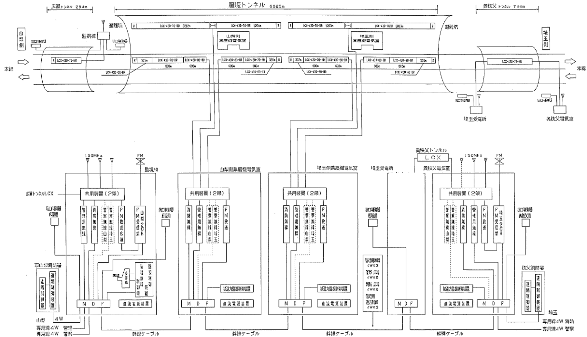
雁坂トンネル無線通信補助設備システム系統図
