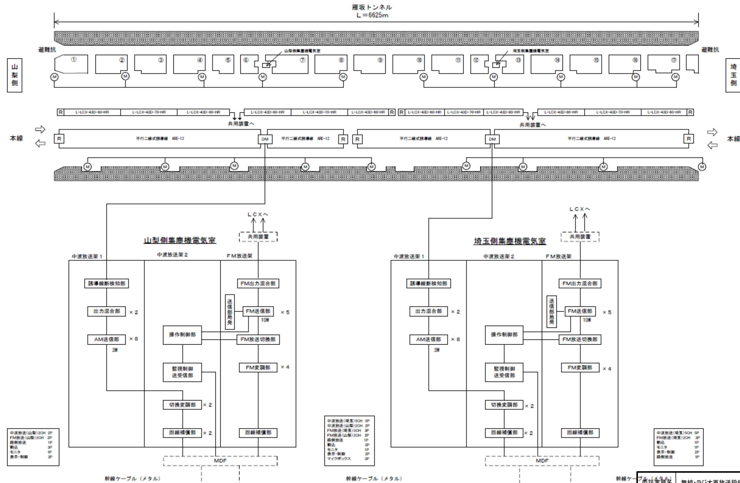
雁坂トンネル ラジオ再放送設備構成図
