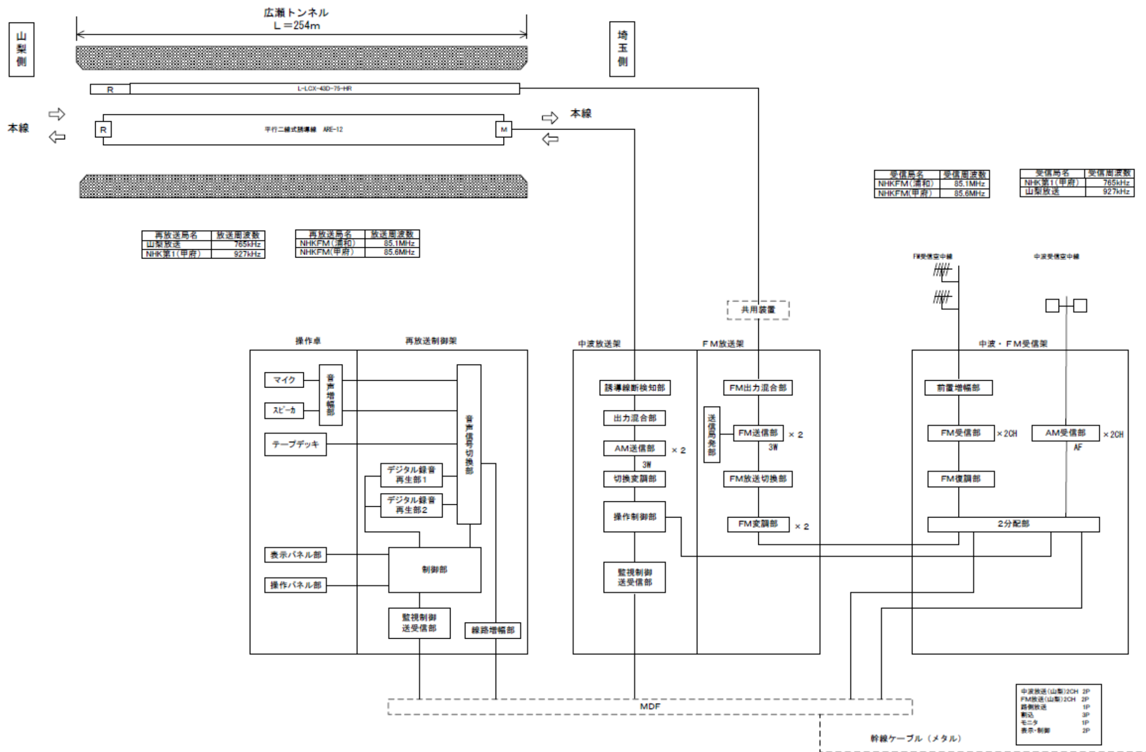
広瀬トンネル ラジオ再放送設備構成図
